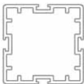
Querschnitt 75 x 75 mm
